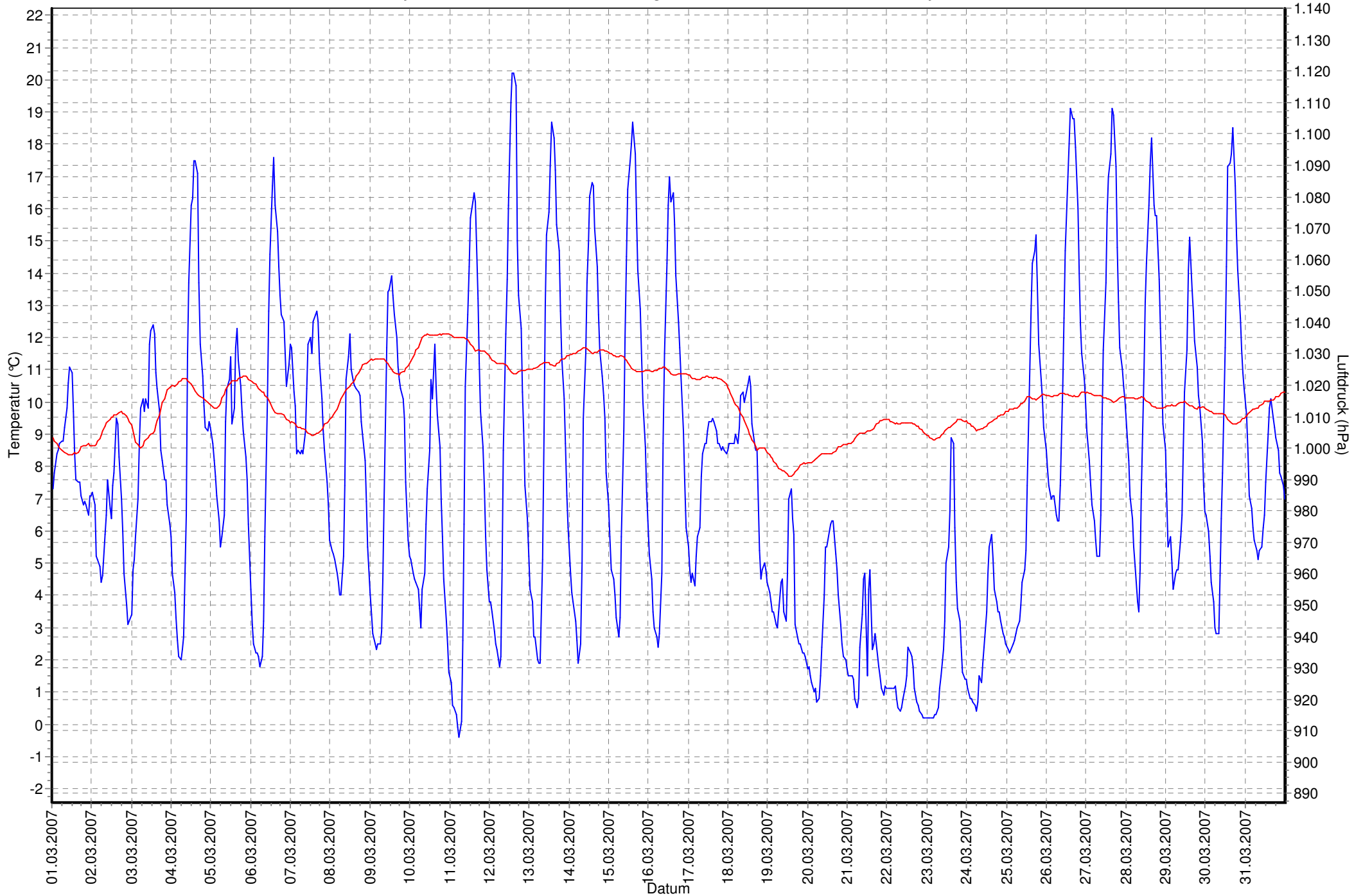
— Aussentemperatur (Y1) — Luftdruck Relativ (Y2)
